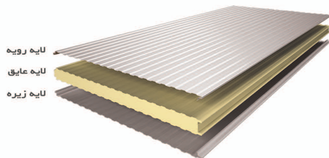
لایه عایق ساندویچ پانل :
